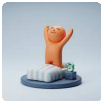
起きる okiru
